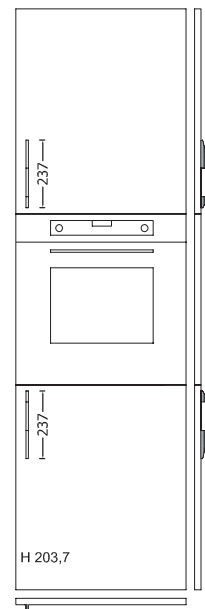
COLONNA FORNO COLUMN OVEN
